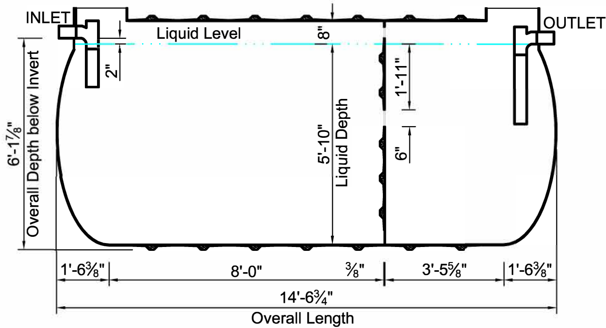
Longitudinal Section
