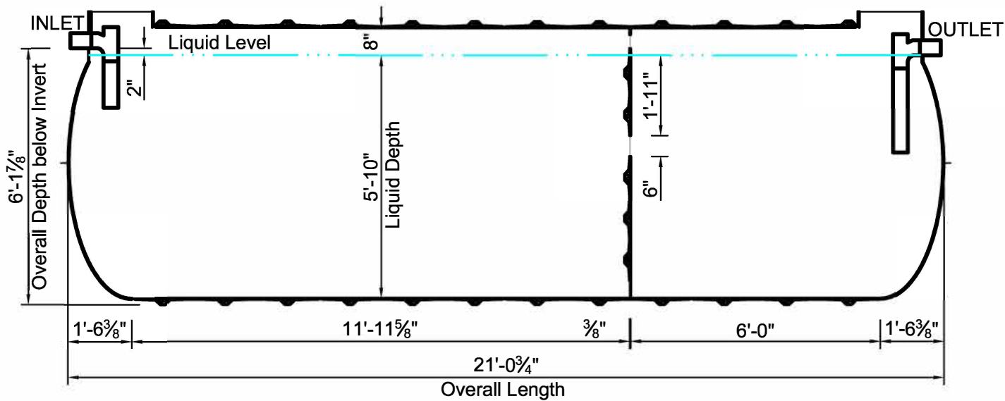
Longitudinal Section
