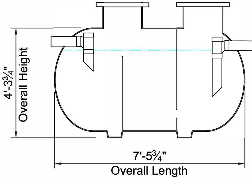
Longitudinal Section
